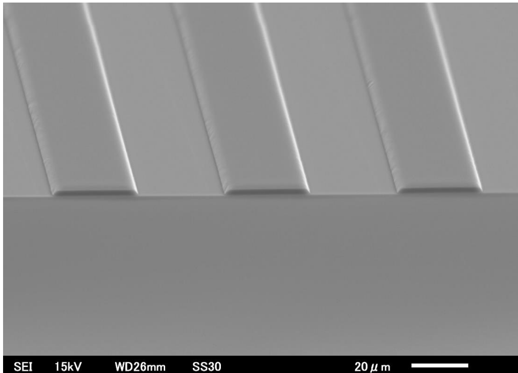
標準ポジレジスト (OFPR-800)
