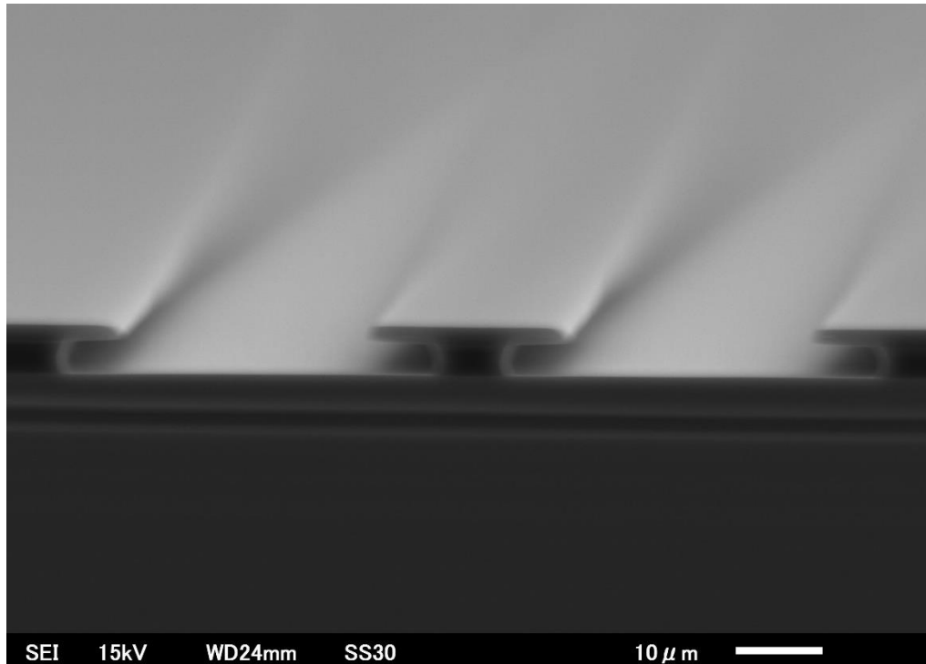
2層レジスト (LOR30B)
