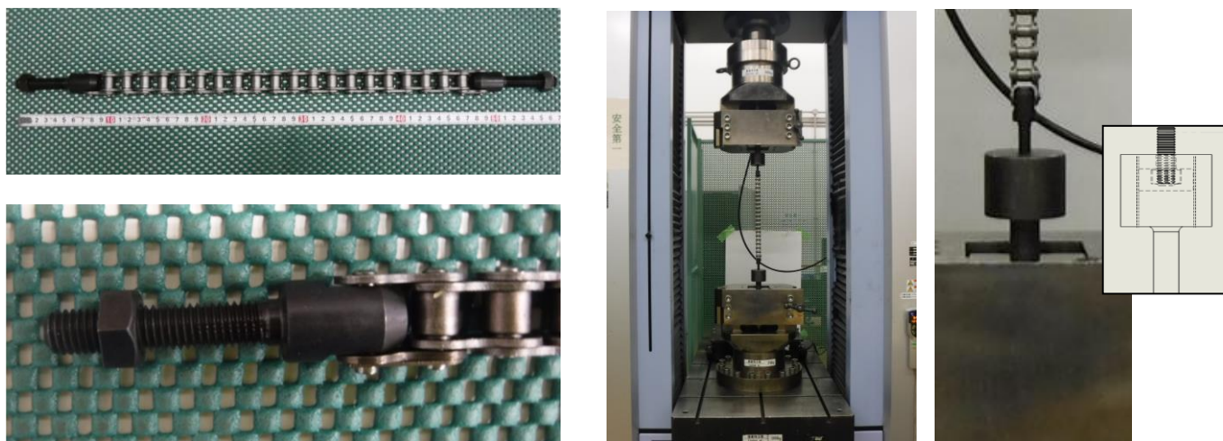
図 1 試験の様子
