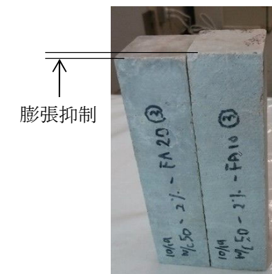
混合材添加による膨張劣化の抑制
