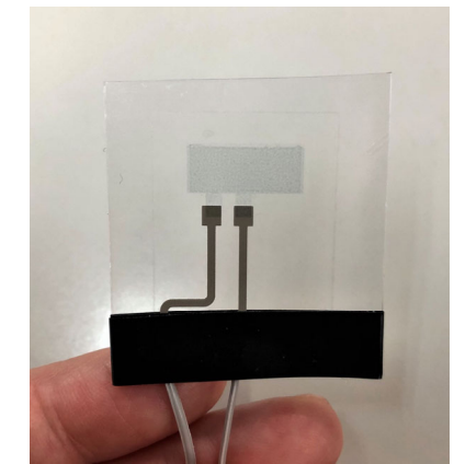
スクリーン印刷技術を用いて作成したフレキシブル圧電センサー
