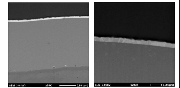
ナノ薄膜材料の断面電子顕微鏡像
