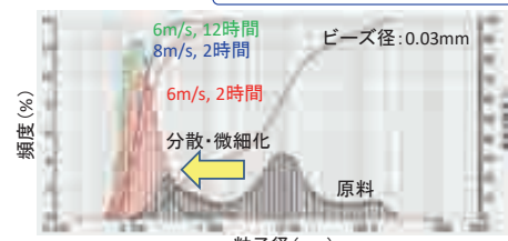
図3 ビーズミル前後の粒度分布
