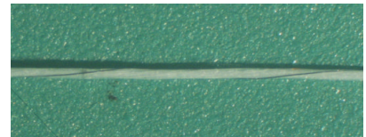
図2 撚糸品 7.5倍拡大 (SUS304 30\mu\text{m} 撚数:300回)
