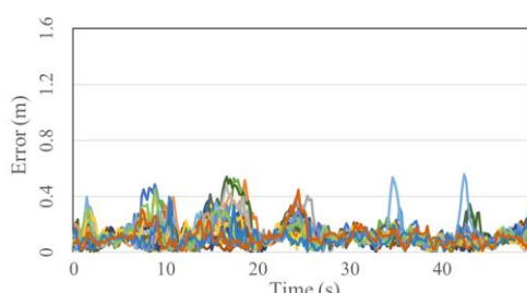
図3 自律移動シミュレーションを20周分行った時の自己位置推定の誤差
