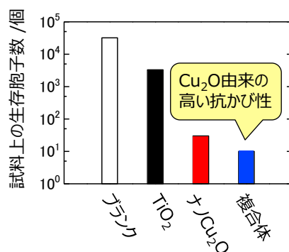
図4 暗所静置18時間後のかび胞子数
